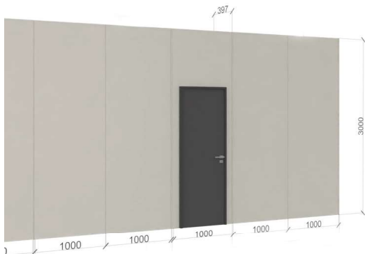
AUSFÜHRUNG Tür mit Blockzarge
