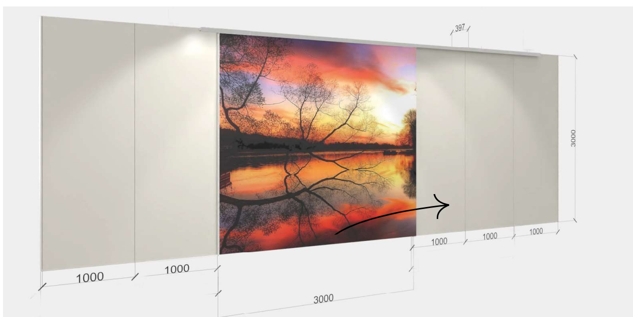
AUSFÜHRUNG der SCHIEBETÜR Breite 3000mm, Höhe 3000mm
